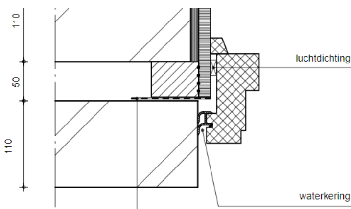
Tekening 11.B4.04
